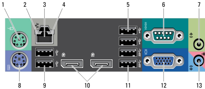
Kuva 3. Minitorni- ja työpöytä tietokoneen takapaneeli
