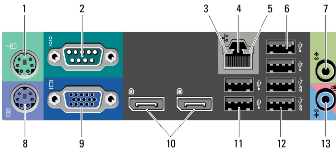
Kuva 5. Pienen kotelon takapaneeli
